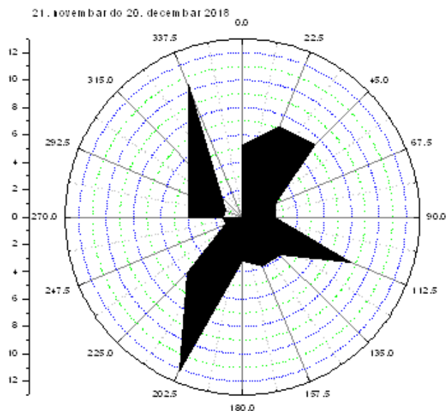
Слика 1. Графички приказ руже ветрова за период узорковања од 21.11. до 20.12.2018.
