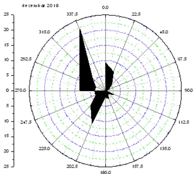
Слика 2. Графички приказ руже ветрова за период узорковања од 01.12. до 31.12.2018.
