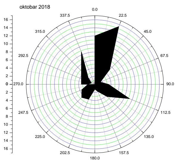
Слика 2. Графички приказ руже ветрова за период узорковања од 01.10. до 31.10.2018.
