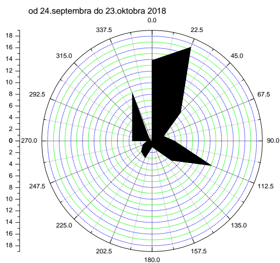
Слика 1. Графички приказ руже ветрова за период узорковања од 24.09. до 23.10.2018.
