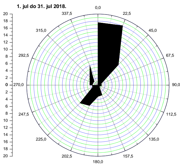
Слика 2. Графички приказ руже ветрова за период узорковања од 01.07. до 31.07.2018.
