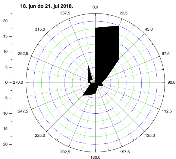
Слика 1. Графички приказ руже ветрова за период узорковања од 18.06. до 21.07.2018.
